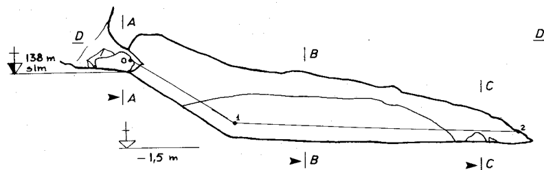
SEZIONE LONGITUDINALE
